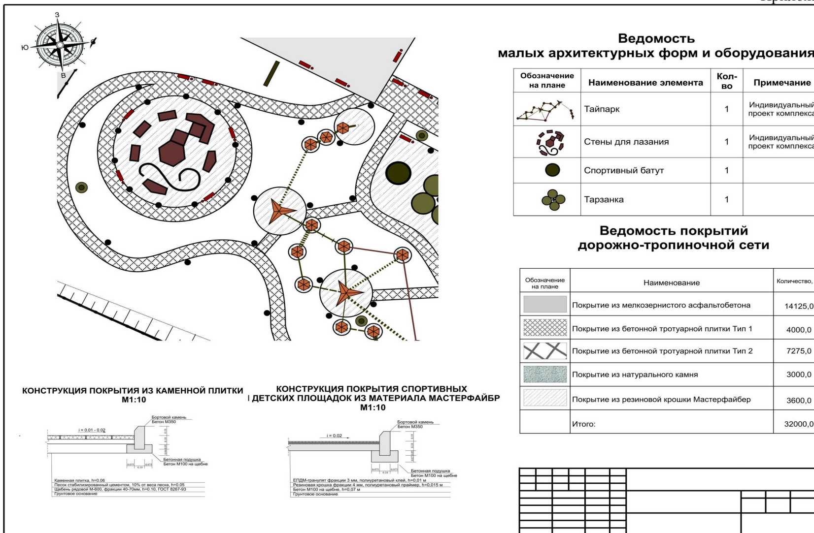
План покрытий дорожно - тропиночной сети и благоустройства территории
