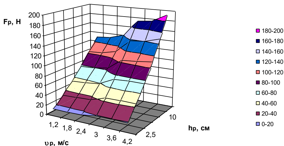
Рис. 5. Изменение сопротивления обработки почвы культиватора с право- и левосторонними плоскорежущими лапами от глубины обработки почвы и скорости движения агрегата
